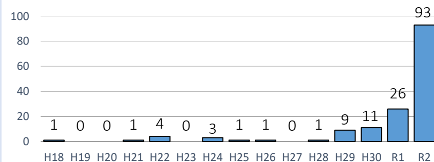
年度別飛来個体数
